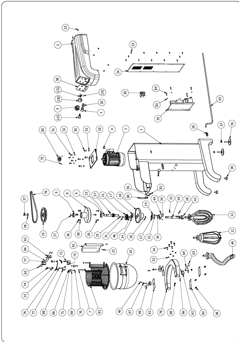
FIG. 33 MP20V Parti ricambio / Replacement parts / Pièces de rechange / Repuestos
